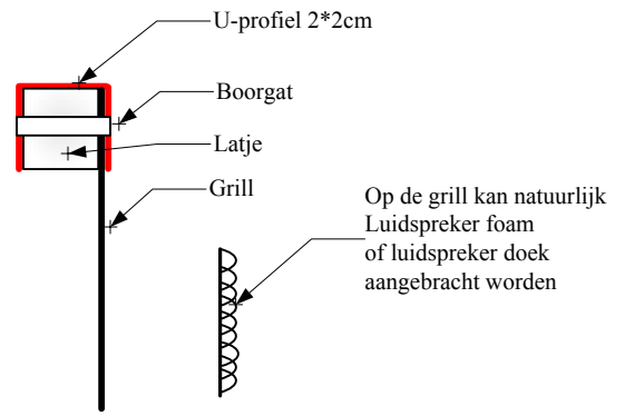
dwars doorsnee
