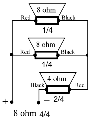
Serie-parallel schakeling van 3 speakers
