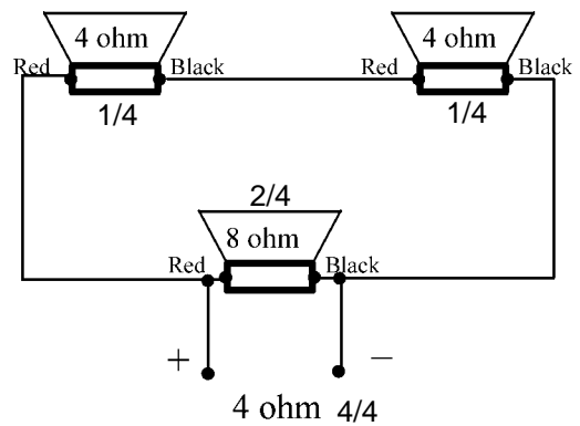
Serie-parallel schakeling van 3 speakers
