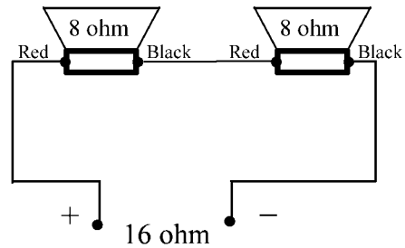
Serie schakeling van 2 speakers
