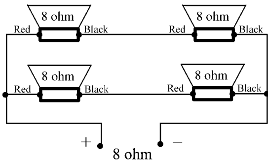
Serie-parallel schakeling van 4 speakers
