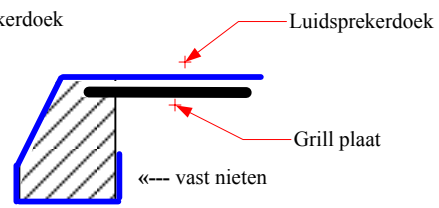
zij aanzicht lat met grill en speakerdoek bekleding lat 4*5cm
