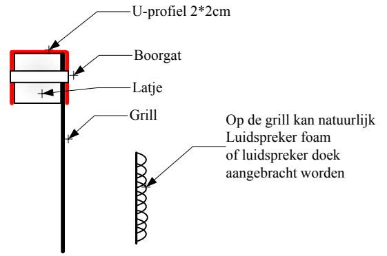
dwars doorsnee
