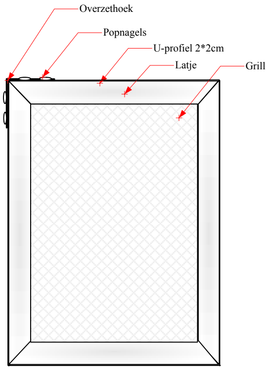
Achter aanzicht
